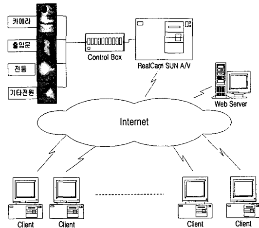
<그림 1> 다목적 실시간 영상/음성 전송 시스템 구성도
