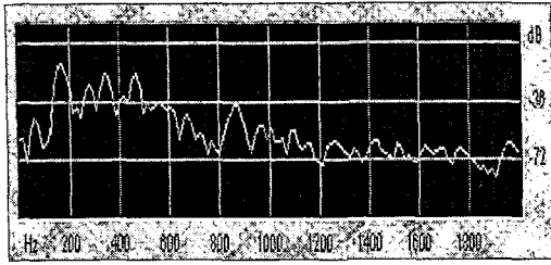
그림 4-2. 에밀레 종소리의 주파수 스펙트럼
