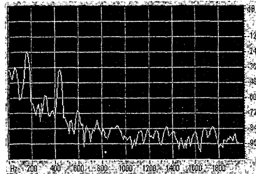
그림 5-1. 백련사 종소리의 주파수 스펙트럼
