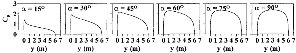
그림 4. 예제구조물의 압력계수 분포형상
