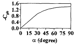
그림 3. 평판상부의 압력계수
