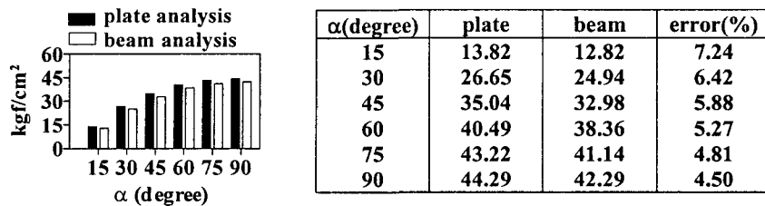
그림 12. 예제구조물 중심부에서의 최대 주응력 비교
