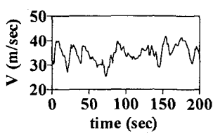
그림 2. 예제바람의 제원
