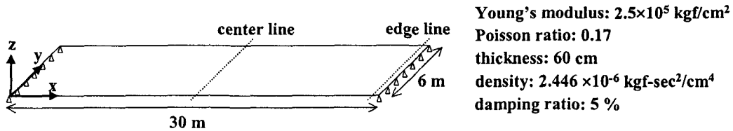
그림 1. 예제구조물의 제원
