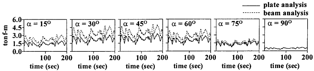
그림 9. 예제구조물 단부에서의 비틀림모멘트 시간이력
