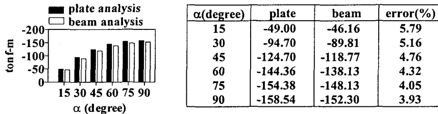
그림 8. 예제구조물 중심부에서의 최대 휨모멘트 비교
