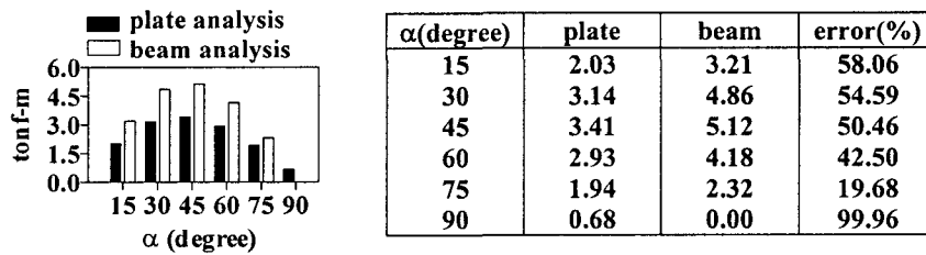
그림 10. 예제구조물 단부에서의 최대 비틀림모멘트 비교
