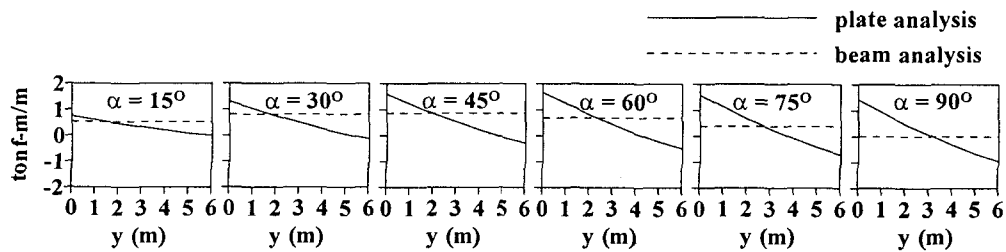
그림 13. 예제구조물 중심부에서의 분포 휨모멘트(time = 154 sec)
