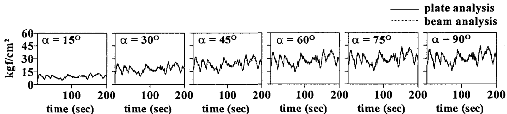
그림 11. 예제구조물 중심부에서의 주응력 시간이력
