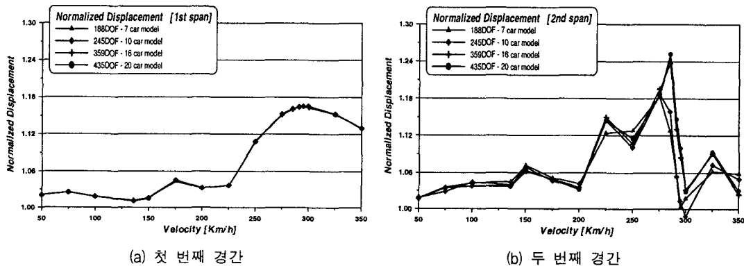
그림 6. 편성모형에 따른 각 경간의 처짐에 대한 증폭계수 비교
