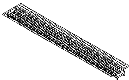
그림 3. 대상교량의 모형화
