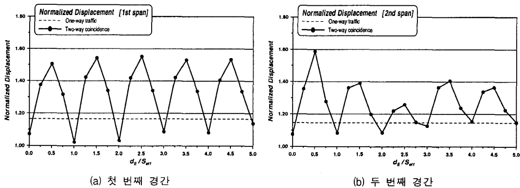
그림 8. 진입거리에 따른 각 경간의 처짐에 대한 증폭계수 비교
