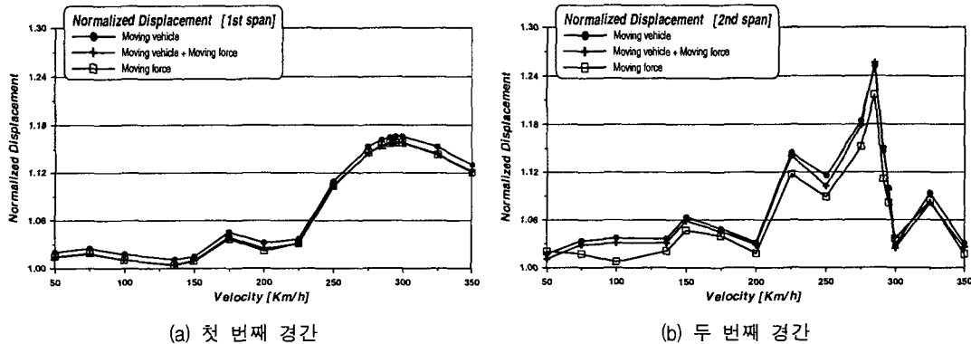
그림 7. 하중모형에 따른 각 경간의 처짐에 대한 증폭계수 비교
