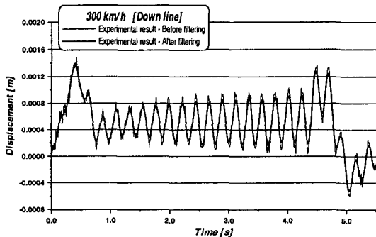
그림 1. 하행시 300km/h의 시간이력곡선
