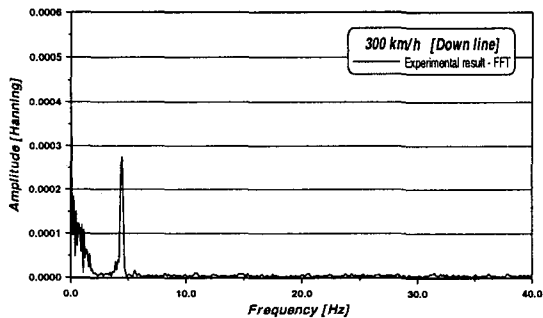
그림 2. 하행시 300km/h의 동적처짐에 대한 스펙트럼
