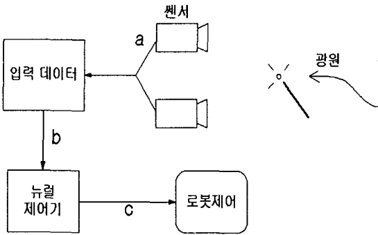
그림 5. 제어구조
