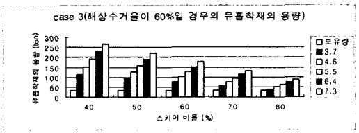
<그림 4-5> 유흡착재의 필요량(CASE 3)
