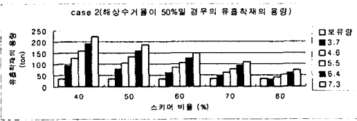
<그림 4-3> 유흡착재의 필요량(CASE 2)
