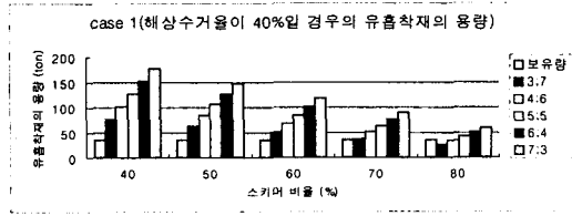
<그림 4-1> 유흡착재의 필요량(CASE 1)
