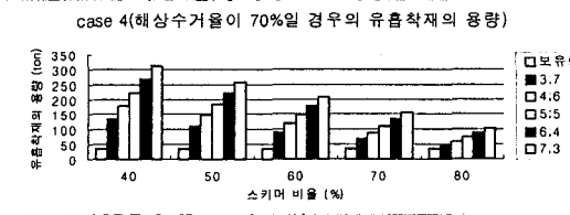
<그림 4-7> 유흡착재의 필요량(CASE 4)
