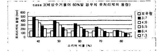
<그림 4-6> 유처리제의 필요량(CASE 3)
