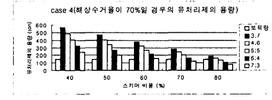
<그림 4-8> 유처리제의 필요량(CASE 4)
