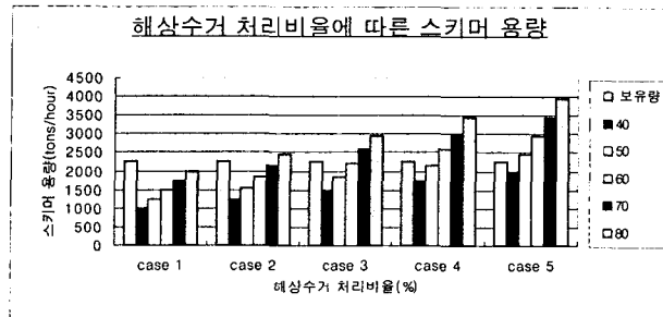
<그림 4-11> 각 CASE 별 스키머의 필요용량
