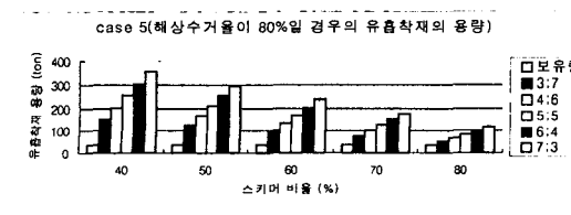
<그림 4-9> 유흡착재의 처리량(CASE 5)
