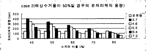
<그림 4-4> 유처리제의 필요량(CASE 2)
