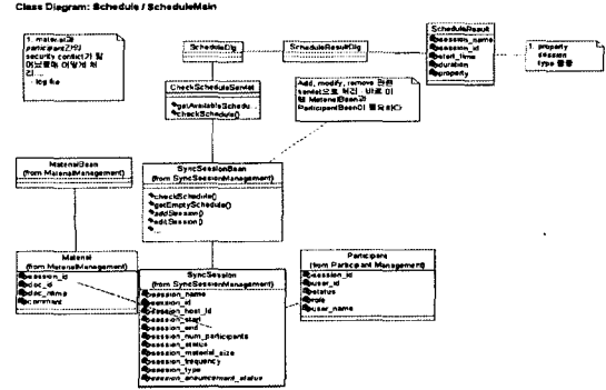
<그림 5> 빈들의 클래스 다이어그램
