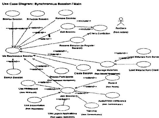
<그림 4> 협업 시스템의 Use Case Diagram
