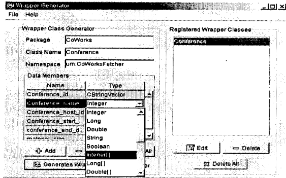
<그림 6> Wrapper Class Generator를 이용하여 객체를 생성하는 예
