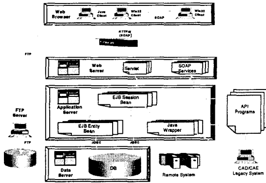
<그림 3> 협업 지원 시스템의 하부구조
