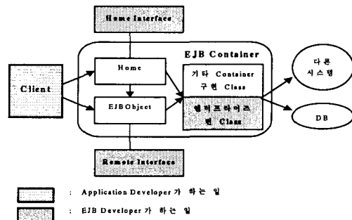
<그림 2> EJB 컴포넌트의 동작
