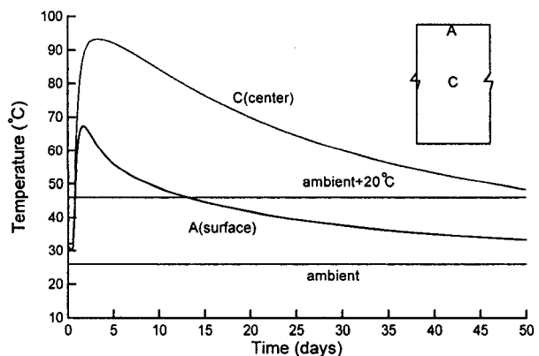
그림 2 매트기초의 온도이력곡선(파이프 쿨링 미적용)
