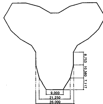
그림 3 매트기초의 형상
