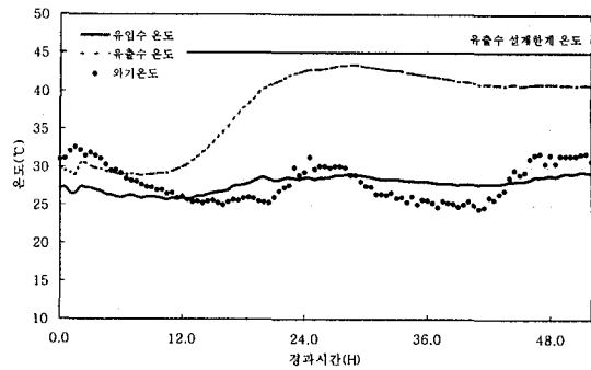
그림 5 측정된 유입수 및 유출수의 온도
