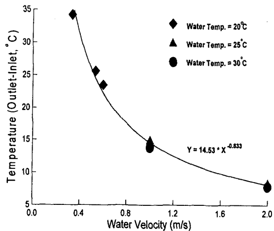
그림 5 1차 통수 중단시 유속과 냉각수 온도차와의 관계
