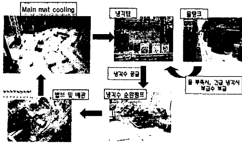
그림 4 Closed loop pipe cooling system
