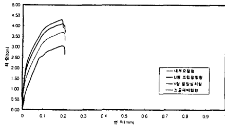
그림 15 전단강도시험의 하중,변위 곡선 (실리카흙)
