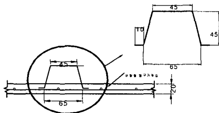
그림 2 U형 조립철망
