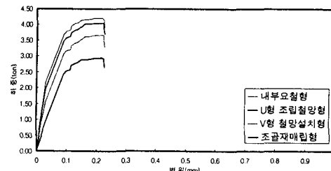
그림 16 전단강도시험의 하중,변위 곡선(플라이애쉬)
