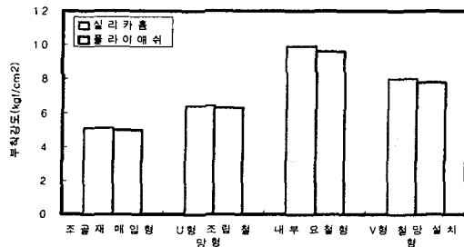
그림 13 영구거푸집의 부착강도 시험 결과
