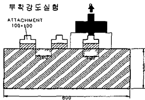
그림 5 부착강도 시험체
