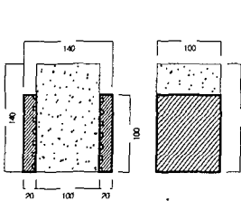
그림 7 전단 시험체
