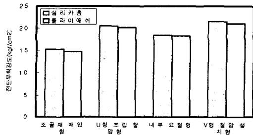
그림 14 전단강도 시험 결과
