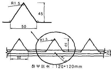
그림 4 V형 철망 설치형
