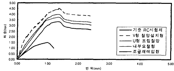
그림20 휨 시험체의 하중 및 변위 곡선(실리카흄 시험체)
