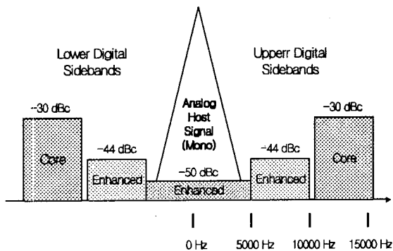
그림 3. 혼성 MF 모드의 IBOC DSB 전력 스펙트럼 밀도
