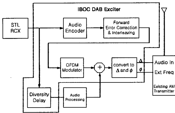
그림 5. 혼성 MF 모드의 IBOC DSB 송신기 블록 다이어그램
