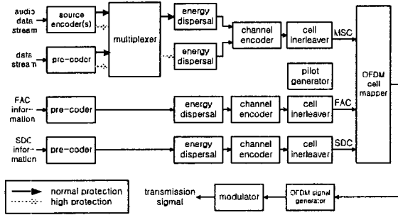
그림 1. DRM 송신기의 블록 다이어그램
