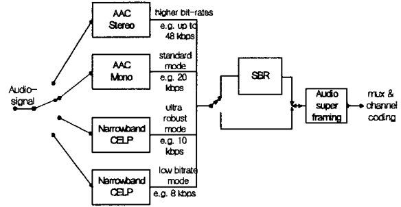
그림 2. 소스 코딩 개념도
