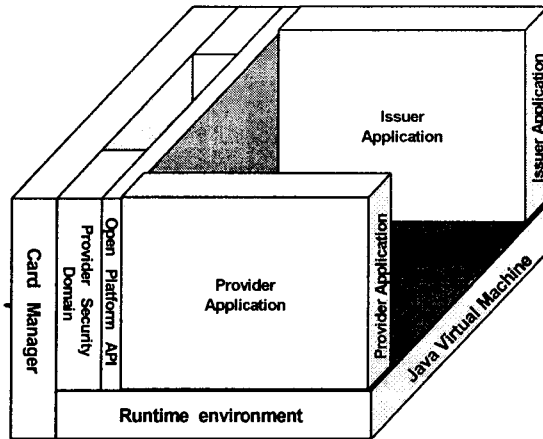
그림 4 : 개방형 플랫폼 구조
