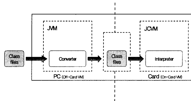
그림 3 : 분리 가상머신 구조
