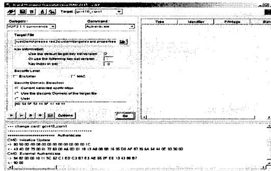
그림 11 : Authenticate
