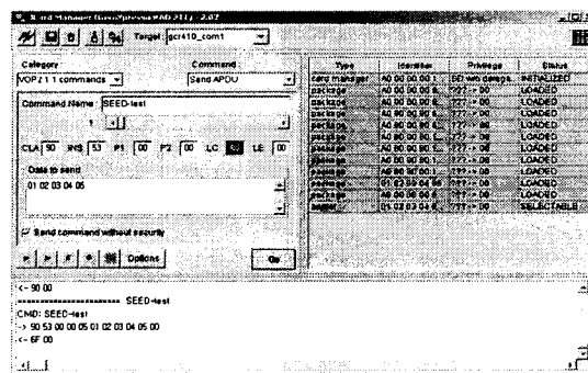
그림 15 : Send APDU
