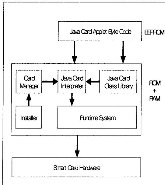
그림 5 : 자바카드 가상머신 구조도
