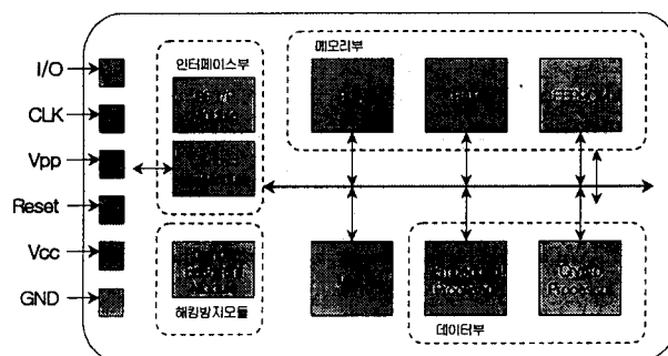
그림 1 : 자바카드의 하드웨어 구조
