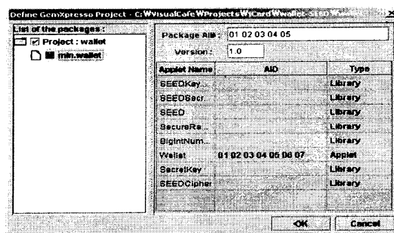
그림 7 : Define Project
