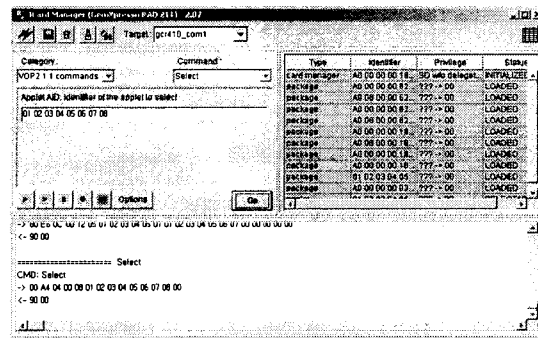
그림 14 : Select
