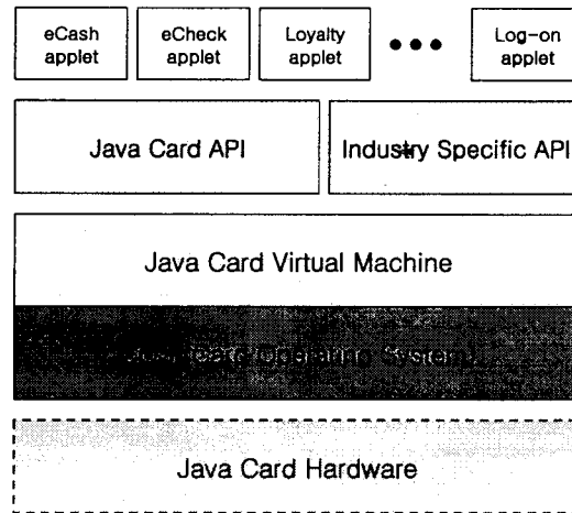
그림 2 : 자바카드 소프트웨어 구조
