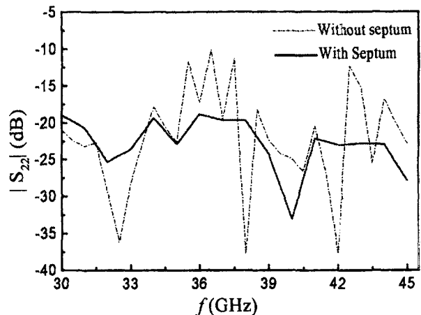
그림 6. 포트 2의 반사손실
