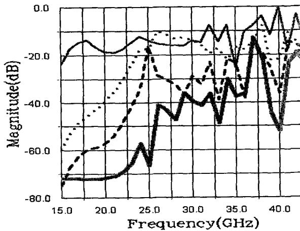
그림 7. 설계된 OMT 의 (a)반사계수, (b)결합계수 가는 실선 : 포트3,4, 가는 점선 : 포트3-2(수평), 굵은 실선 : 포트3-2(수직), 굵은 실선 : 포트2(수평)-2(수직)
