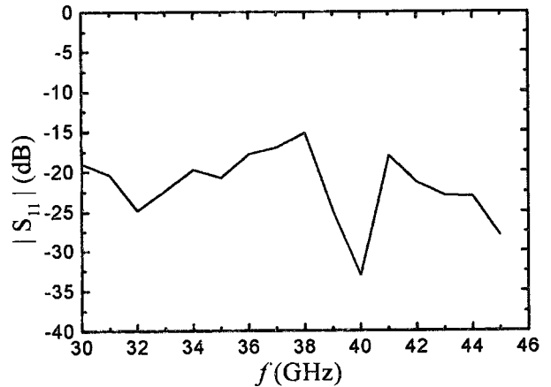
그림 3. 정사각형-정사각형 도파관 변환부 특성
