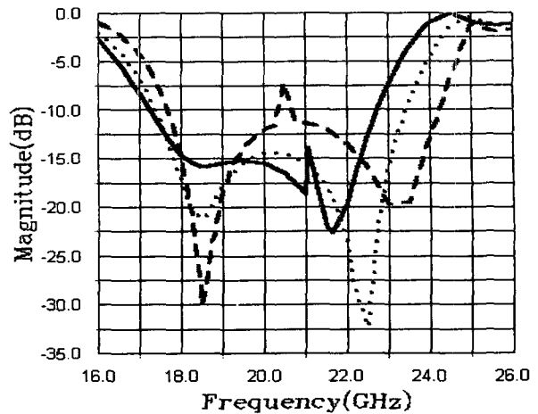
그림 5. 측면포트 결합슬롯 위치에 따른 반사특성. 실선: G_4=0.7\text{ mm} , 점선: G_4=0.3\text{ mm} , 쇠선: G_4=1.3\text{ mm}
