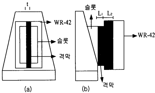
그림 2. 측면 포트에 격막이 삽입된 모양 (a) 정면도 (b) 측면도
