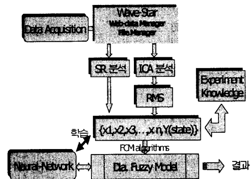
그림 9. 절연열화 진단시스템의 블록 다이어그램 Fig. 9. Block-Diagram of Insulation Degradation Diagnosis System
