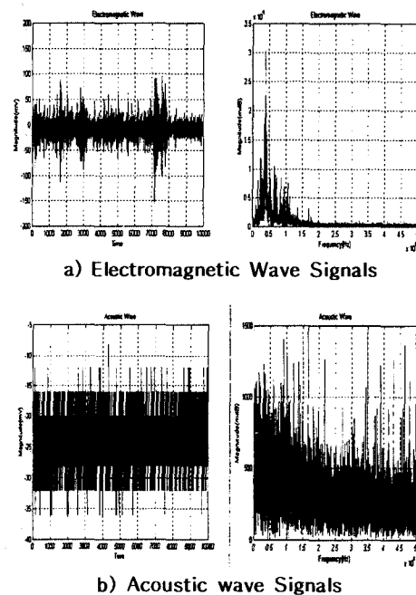
그림 2. 전자파와 초음파신호의 데이터 Fig. 2. Row Data of Electromagnetic and Acoustic Wave signals
