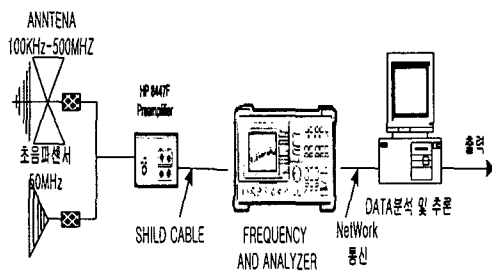
그림 1. 전자파 및 초음파 측정장치 Fig. 1. Composition of Electromagnetic and Acoustic measurement system
