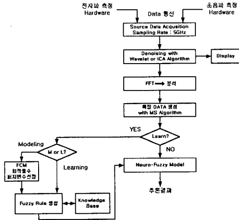
그림 10. 진단 알고리즘 흐름도 Fig. 10. Flowchart of Diagnosis Algorithms
