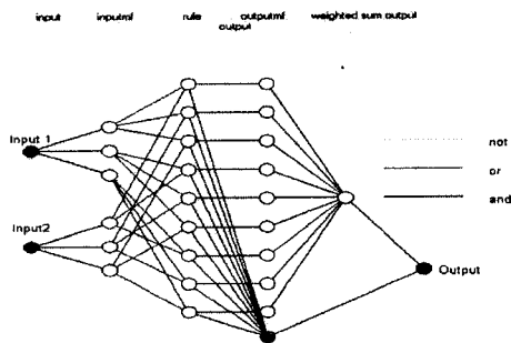
그림 11. 학습된 뉴로-퍼지 모델 Fig. 11. Learned Neuro-Fuzzy Model
