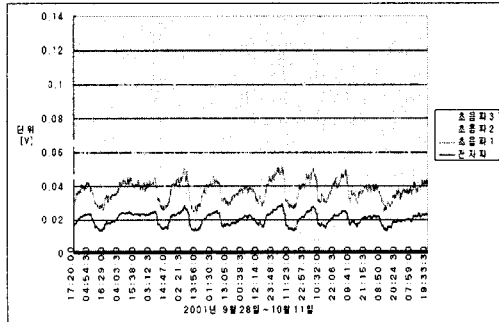
그림 3. 이동평균 후 트렌드 Fig. 3. Trend after Moving Average
