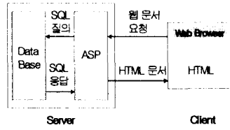
<그림 1> ASP를 이용한 동적 구동원리
