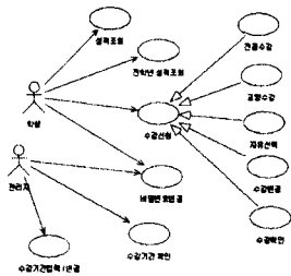
<그림 2> 본 시스템의 Usecase Diagram
