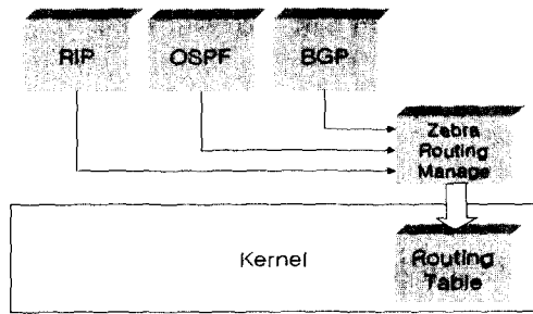
[그림 1] Zebra의 구조
