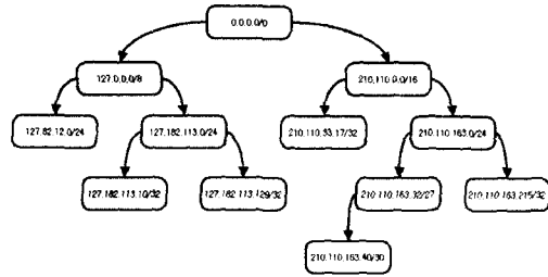
[그림 3] 라우팅 테이블의 구성 예
