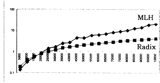
[그림 4] 생성시간 과 추가 IP 수
