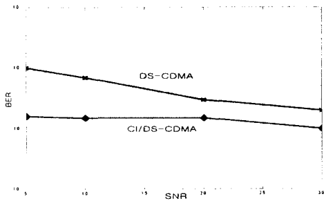
그림 8 SNR에 대한 BER(이용자 30명). Fig.8. BER vs SNR for 30 users.
