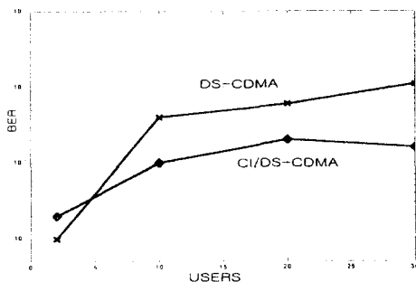
그림 9 이용자수에 따른 BER(SNR 5dB). Fig.9. BER vs users for SNR 5dB.
