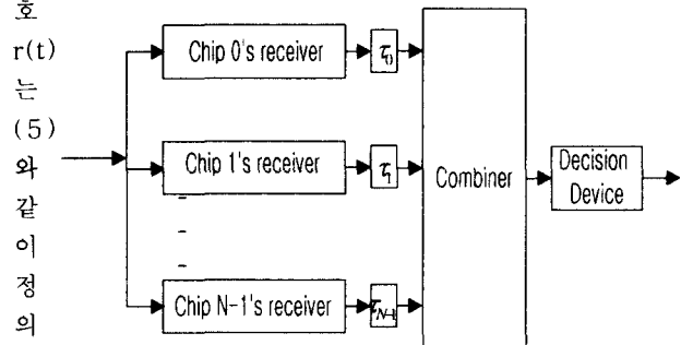
그림 2. 수신기 구조. Fig.2. Receiver structure.
