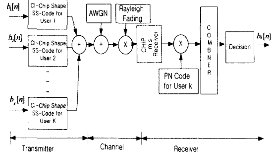
그림 4 CI/DS-CDMA 시뮬레이션 구성도 Fig.4. Block diagram for CI/DS-CDMA simulation
