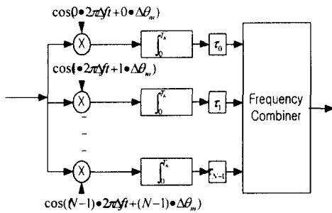
그림 3. m 번째 칩 수신기. Fig.3. The mth Chip receiver.
