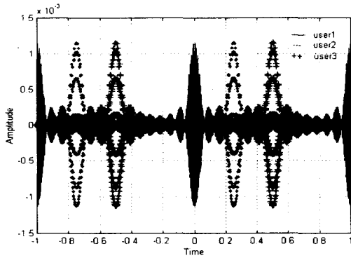
그림 7. 3명의 이용자를 위한 CI 신호. Fig.7. CI signals for 3 users.
