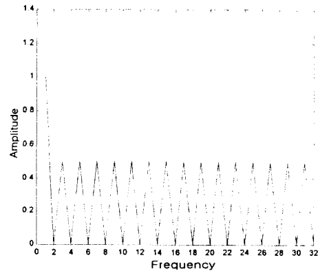
그림 6. CI 신호의 FFT. Fig.6. FFT of CI signals. 은 CI 필터 h(t) 를 이용하여 발생되며 SS(Spread
