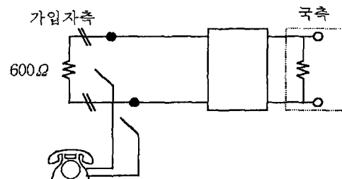
그림 5. 측정회로(일본)
