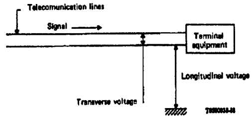
그림 2. 유도 전압 모드
