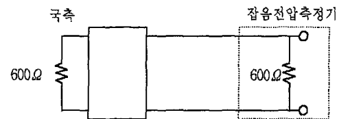
그림 4. Bellcore 측정회로
