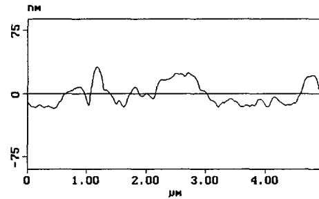
그림 5. LB막의 roughness
