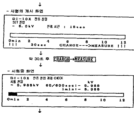
그림 4. 잔류전압 측정화면 Fig. 4. Picture of residual voltage test
