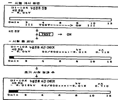
그림 2. 직류누설전류 시험중 화면 Fig. 2 Picture during insulation resistance test
