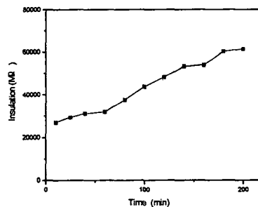
그림 7 측정 시간과 절연 저항과의 비교 Fig. 7. Relation between measuring time and insulation resistance
