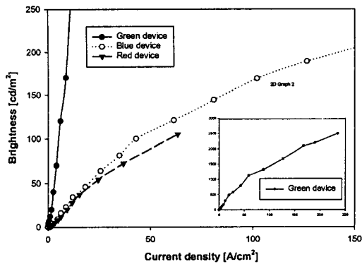
그림 5 전류밀도와 휘도와의 관계 (● 녹색 소자 ○ 청색 소자 ▼ 적색 소자) Fig. 5. The relation of current density and brightness. (● green device ○ blue device ▼ red device)
