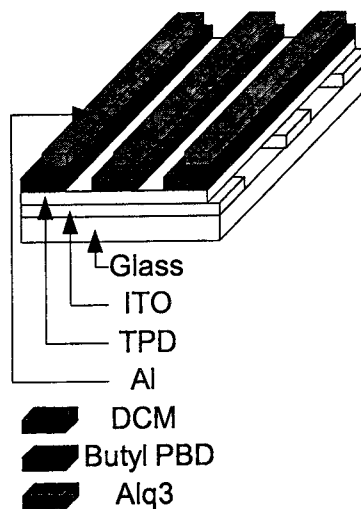
그림 2 삼원색 유기 발광 소자의 구조
