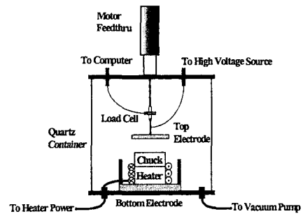
그림 1. 고착압력 측정장치의 도식도
