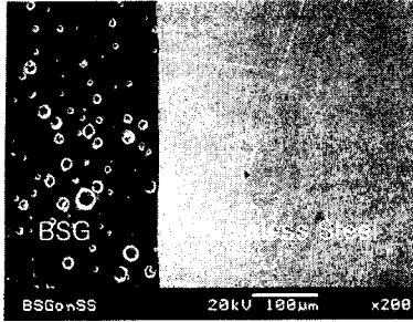
그림 2. 소다붕규산염 유리/스테인레스스틸 계면에서의 주사전자현미경 미세조직.
