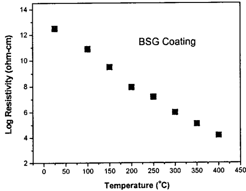
그림 5. 온도변화에 따른 소다붕규산염 유리의 전기비저항.
