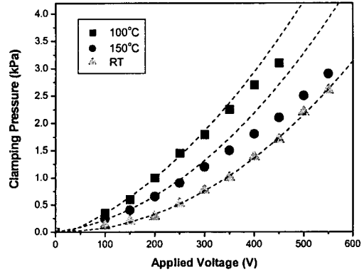
그림 3. 온도에 변화에 따른 소다붕규산염 유리/스테인레스스틸 ESC의 고착압력.
