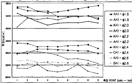
[그림 3] 관경별 휘도 분포
