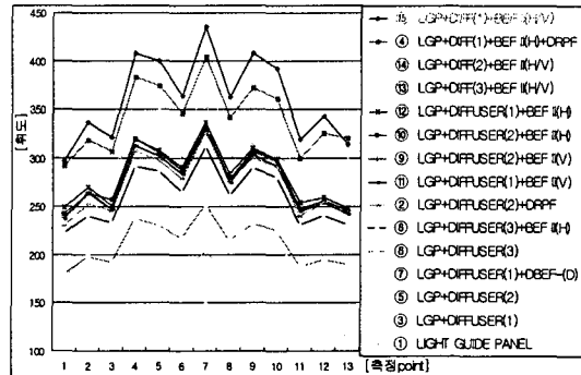
[그림 5] 시트 Variation에 따른 휘도 분포
