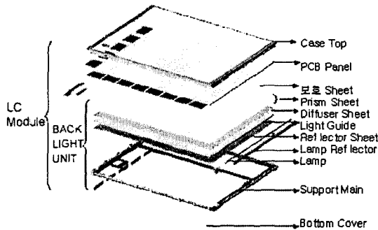
[그림 1] BLU 구조
