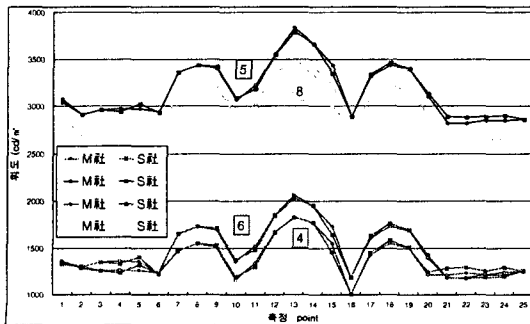
[그림 4] 두께별 휘도 분포
