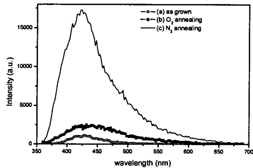
그림 1. He 1 Torr에서 증착 후 (a) 후열처리하지 않은 Si 박막, (b) 산소 및 (c) 질소분위기에서 760 °C에서 10분간 후열처리한 박막의 PL 스펙트럼.
