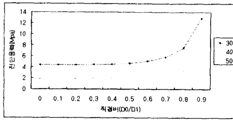
그림 4. 직경비에 따른 전단응력
