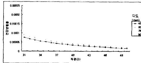
그림 7. 직경과 각도에 따른 전단변형률(D/D1=0.4)
