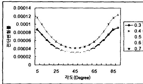
그림 5. 각도와 직경비에 따른 전단변형률( \epsilon_{xy}^0, D=40 )
