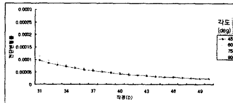
그림 8. 직경과 각도에 따른 전단변형률(D/D1=0.6)
