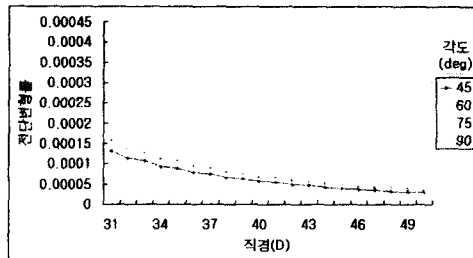
그림 9. 직경과 각도에 따른 전단변형률(D/D1=0.8)
