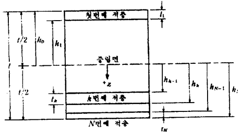
그림. 1 적층판의 형상
