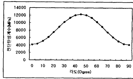
그림 6. 각도에 따른 전단탄성계수
