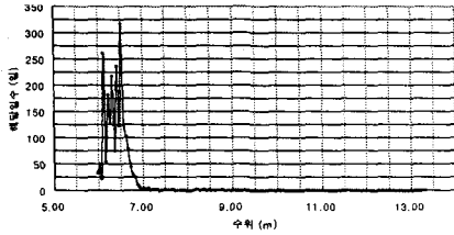
Fig. 3 Suction water level of Jayang pump station(1993~1998년)
