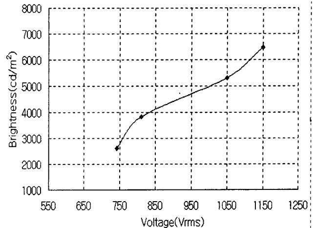
그림 4 전압에 따른 휘도 특성 Fig. 4 Luminance characteristics by voltage.
