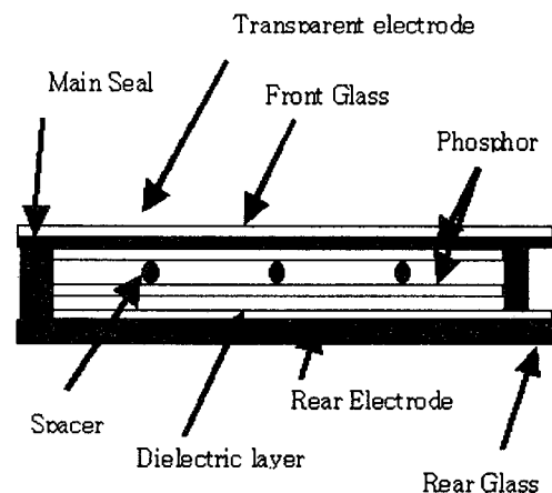
그림 1 램프의 구조 Fig. 1 construction of Lamp
