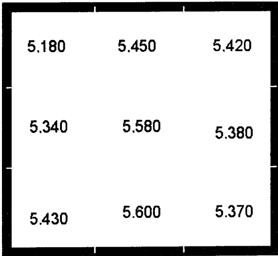
그림 3 램프의 휘도 분포 Fig. 3 Luminance distributed of lamp
