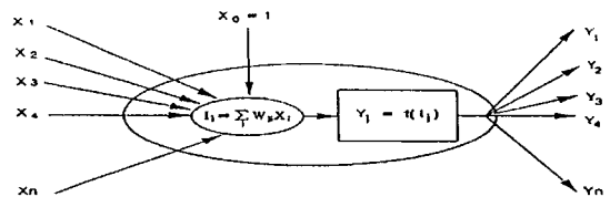
그림 1 뉴런의 모델 Fig. 1 Model of neuron
