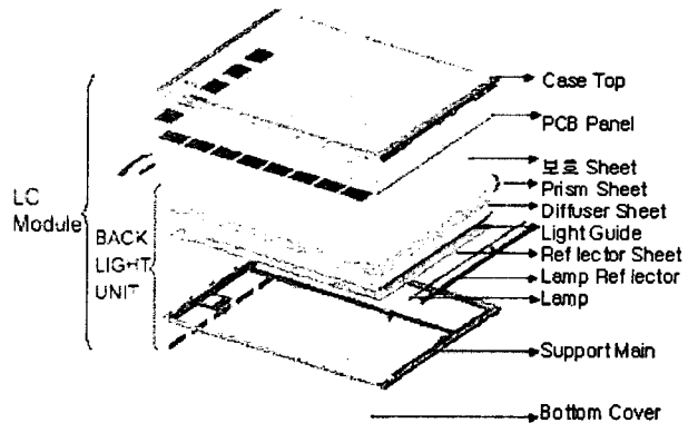
그림 1 BLU 구조
