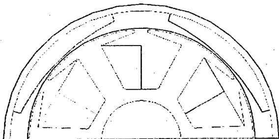
그림 2 BLDC 전동기의 단면도
