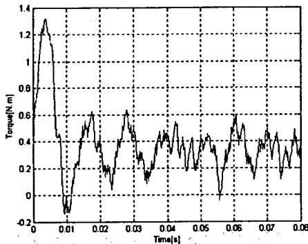
(a) 듀티비가 50%인 경우
