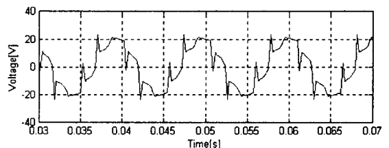
(a) 듀티비가 50%인 경우
