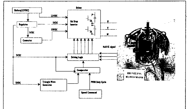
그림 3 BLDC 전동기의 제어 블록 시스템
