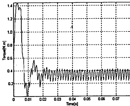
(b) 듀티비가 95%인 경우
