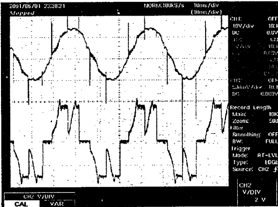
(b) 듀티비가 95%인 경우
