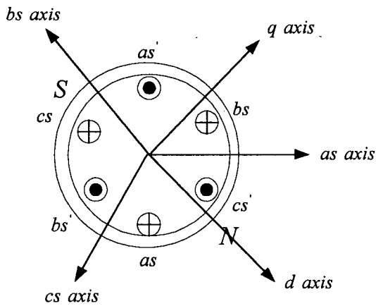
그림 1 BLDC전동기의 벡터도
