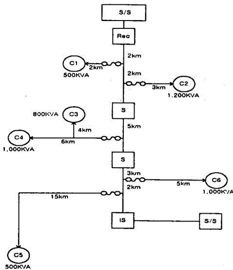
그림 1. 22.9kV 방사상 모델 배전계통
