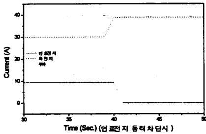
(그림 4) 부하 및 전류 변화에 따른 연료전지의 전압 전류 분포
