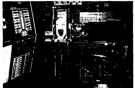
[그림 3] 연료전지 축전지 복합 동력원 구성 장치
