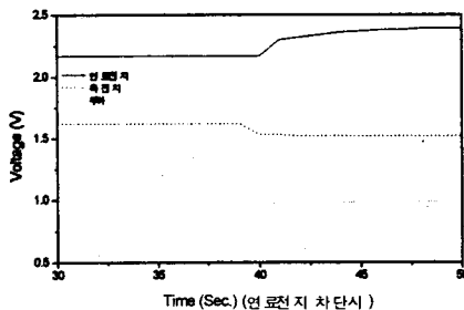
(그림 5) 연료전지의 동력 차단시 축전지 및 부하의 전류 전압 분포
