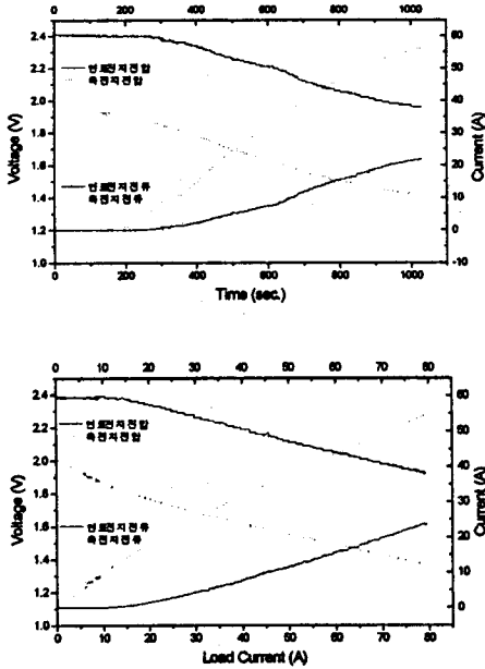
(그림 4) 부하 및 전류 변화에 따른 연료전지의 전압 전류 분포
