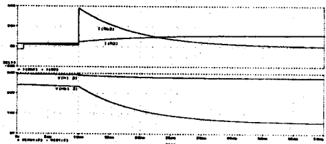
[그림 1] 연료전지 축전지 부하 분담 해석
