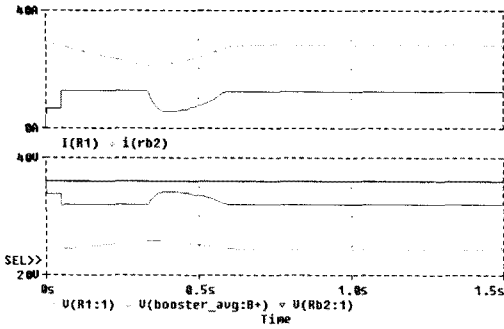
[그림 2] 이득 변화에 따른 출력 특성 변화
