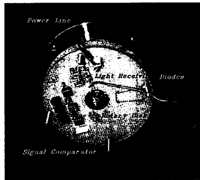
그림 5 제작된 엔코더 Fig.5 Prototype encoder
