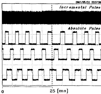
그림 6 SRM 구동시 엔코더의 출력파형 Fig.6 Output waveform of encoder during SRM driving
