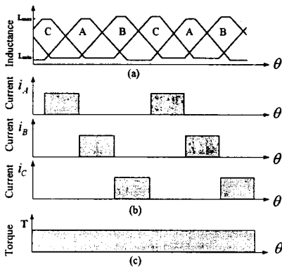
그림 2 6/4 SRM에서 각 상의 인덕턴스 프로파일에 대한 이상적인 상전류 파형과 토크 (a) 인덕턴스 프로파일 (b) 상전류 (c) 토크 Fig.2 Ideal phase current and motoring torque with inductance profiles for 6/4 SRM (a) Inductance profile (b) Phase current (c) Torque
