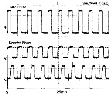
그림 7 엔코더 출력에 따른 게이트신호 Fig. 7 Gate pulse with encoder output
