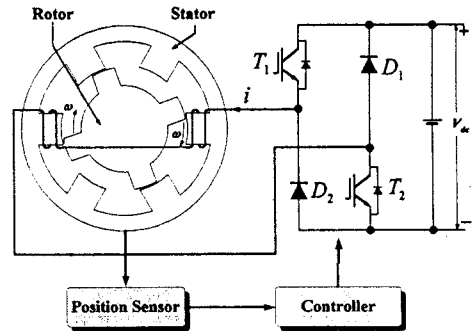
그림 1 SRM 구동시스템 Fig.1 SRM drive system
