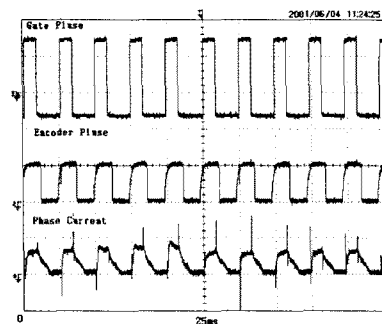
그림 8 한상의 게이트 신호, 엔코더 신호, 상전류 Fig.8 Gate signal, encoder signal and phase current of one phase
