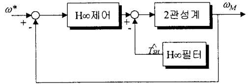
그림 5 H \infty 필터를 이용한 새로운 속도제어
