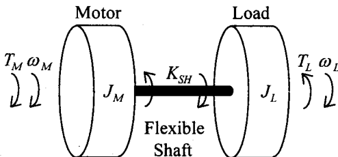
그림 1 2관성계 플랜트 모델
