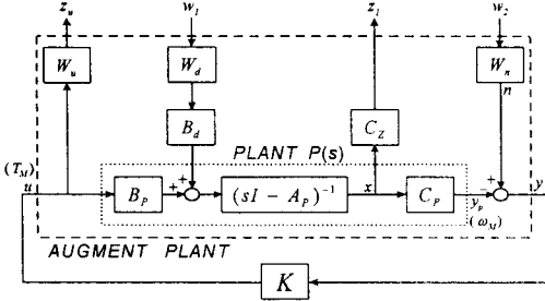
그림 3 H \infty 제어 일반화플랜트
