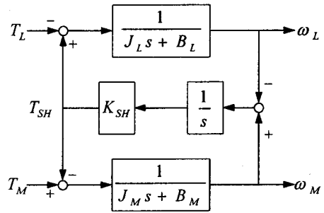
그림 2 2관성계 블럭선도
