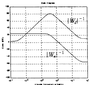
그림 4 가중함수의 보드선도
