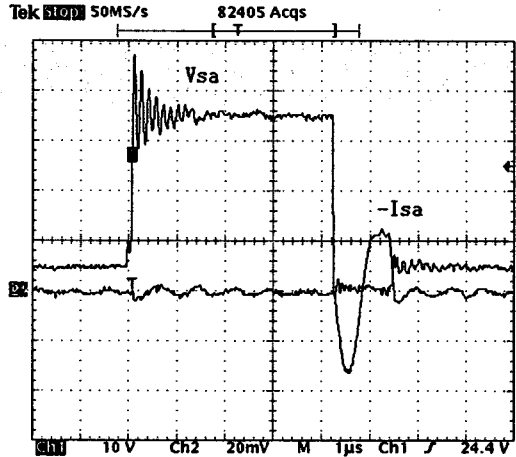
그림 6. 보조 스위치의 전류,전압(2A/div,10V/div)
