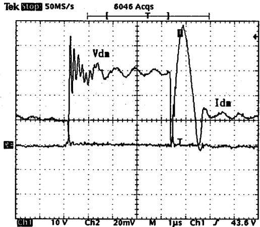
그림 7. 주 다이오드의 전류,전압(2A/div,10V/div)
