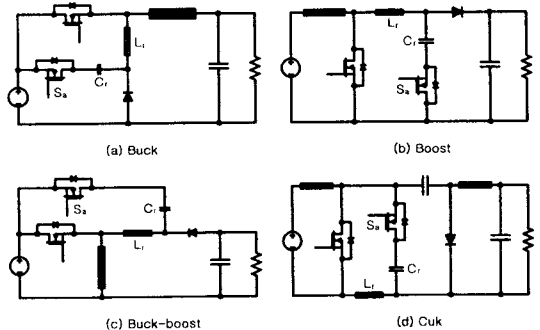
그림 4. 확장된 ZCS-PWM 컨버터 회로
