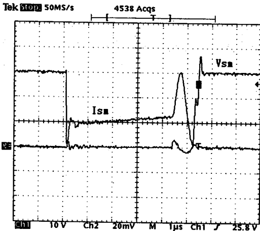
그림 5. 주 스위치의 전류,전압(2A/div,10V/div)
