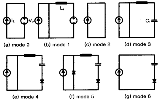
그림 2. 제안된 컨버터의 스위치 모드
