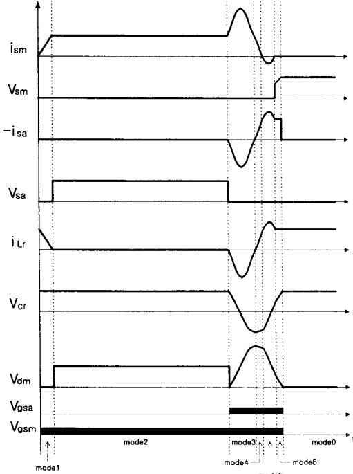
그림 3. 한 주기 동안의 스위칭 파형
