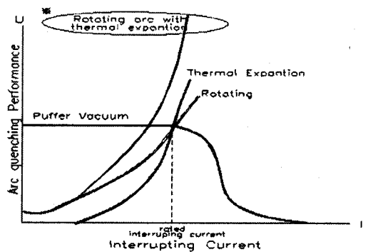
그림 1. 차단 방식별 소호 능력 비교
