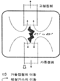
그림 3 열팽창에 의한 아크 소호
