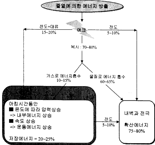
그림 2. 아크에 의한 소호부 에너지 분포도
