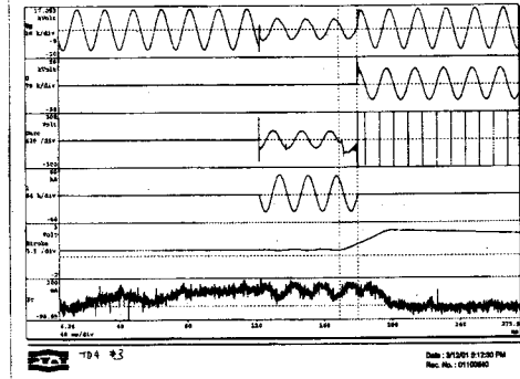
그림 8. 24kV, 25kA TD 4 차단시험 파형
