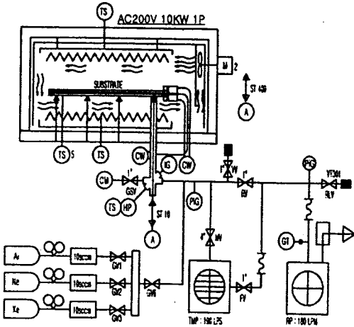
그림 1 블록 다이어그램 Fig. 1 .Block diagram
