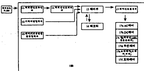
그림 1 적외선 리모콘 송·수신 신호처리 Block Diagram
