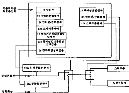
그림 3 인터폰/전화 응용 Block Diagram
