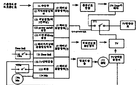
그림 2 도어폰 응용 Block Diagram
