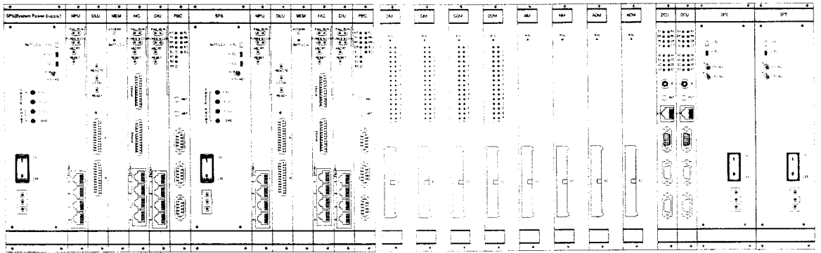
그림 2. MPU 셀프의 외관 및 I/O 셀프의 외관
