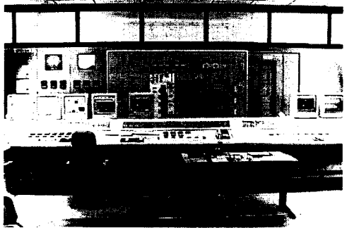
그림 5. 개조후의 호남화력 2호기 중앙제어반
