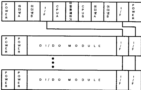
그림 3. BMS 시스템의 현장 제어반 구성도
