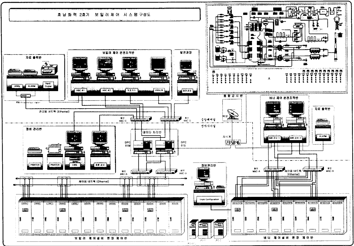
그림 1 국산 개발한 디지털 분산제어시스템 구성도
