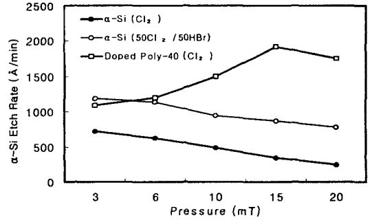
그림 1. 바이어스 전력 0W 및 소스 전력 500W 하에서 반응로 압력에 따른 식각율
