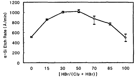
그림 2. 바이어스 전력 0W, 소스 전력 500W 및 반응로 압력 10mTorr 하에서 \text{Cl}_2/\text{HBr} 가스 혼합비에 따른 도핑되지 않은 비정질 실리콘의 식각율
