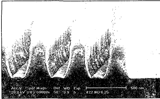
그림 6. 반응로 압력 3mTorr, 소스 전력 300W, 바이어스 전력 30W 및 Cl_2(35)/HBr(35)/O_2(7) 가스 혼합 조건에서 식각한 후, C_2F_6 를 이용하여 게이트 산화막을 제거한 시료의 SEM 단면 사진
