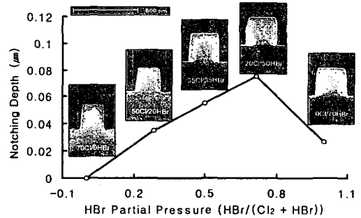
그림 5. 반응로 압력 3mTorr, 소스 전력 300W, 바이어스 전력 30W 및 Cl 2 (X)/HBr(Y)/O 2 (7) 가스 혼합 조건에서 Cl 2 /HBr 가스 혼합비에 따른 격리된 패턴에서의 나침 깊이
