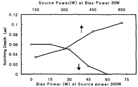
그림 4. 반응로 압력 3mTorr, 소스 전력 300W, 바이어스 전력 30W 및 Cl 2 (35)/HBr(35)/O 2 (7) 가스 혼합 조건에서 소스 전력 및 바이어스 전력의 변화에 따른 격리된 패턴에서의 나침 깊이의 경향성
