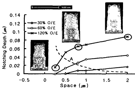
그림 3. 반응로 압력 3mTorr, 소스 전력 300W, 바이어스 전력 30W 및 Cl 2 (35)/HBr(35)/O 2 (7) 가스 혼합 조건에서 과도 식각 시간 및 라인 공간에 따른 나침 깊이의 경향성
