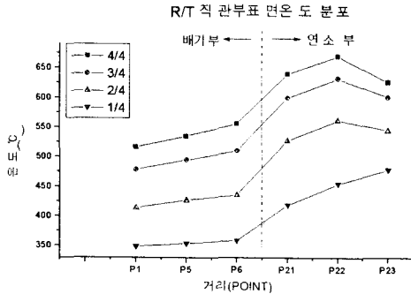
[그림 6] 복사튜브 직관부 표면온도 분포
