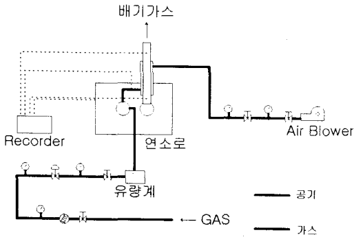
[그림 1] 실험장치도
