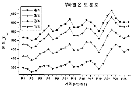
[그림 3] 부하별 복사튜브 표면의 거리별 온도분포
