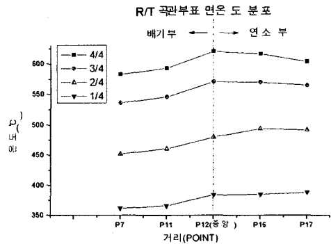
[그림 5] 복사튜브 곡관부 표면온도 분포
