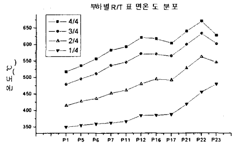
[그림 4] 부하별 복사튜브 표면온도 분포
