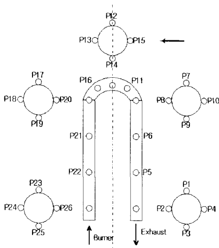
[그림 2] 복사튜브의 온도 측정지점
