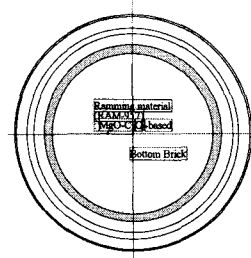
Fig. 1 STS VOD Ladle
