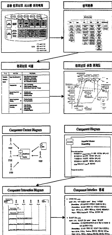
[그림 3.1] 컴포넌트 명세방법
