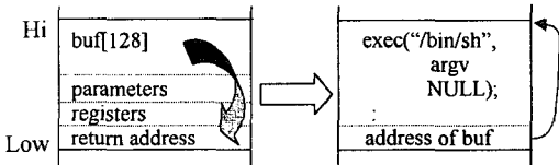
(그림 3) sub2() 스택 프레임의 변화
