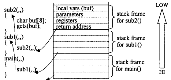
(그림 2) C/C++ 함수호출과 스택변화
