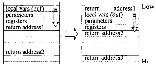
(그림 4) 복귀주소 위치에 따른 버퍼넘침의 영향
