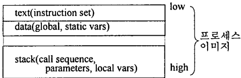
(그림 1) UNIX a.out 포맷
