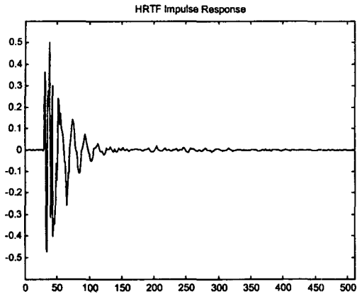
그림 2. FIR 형태의 512탭수의 HRTF의 임펄스응답
