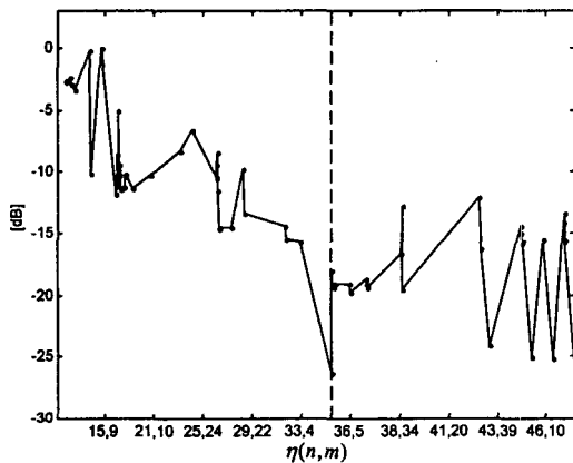
그림 3. 모델차수 선택을 위한 오차값 \eta(n, m)
