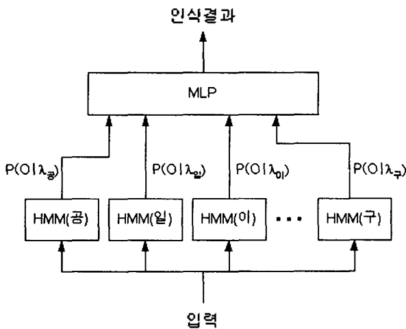
그림 1. HMM과 MLP의 하이브리드 시스템
