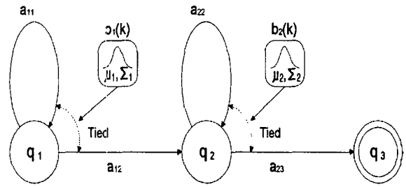
그림 2. 연속 출력확률 HMM
