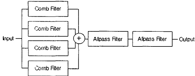
그림 4. 구현된 잔향기
