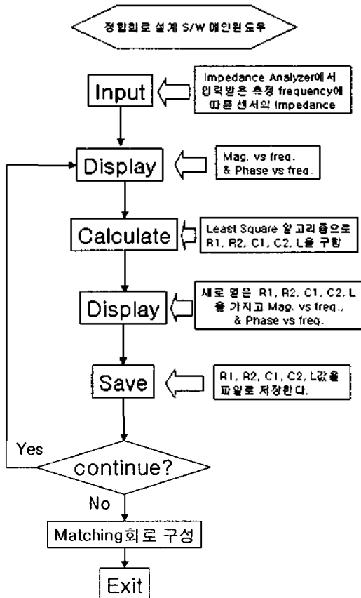
그림 1 정합회로 설계 S/W의 간략한 순서도
