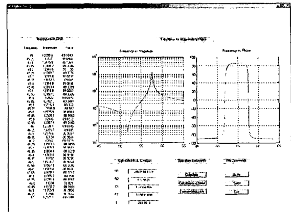
그림 5. 계산 후 R, L, C 값들을 표시한 화면
