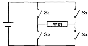
그림 1 인버터의 기본구조
