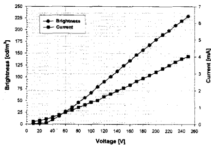
그림 7 인가 전압 변화에 따른 휘도와 전류특성
