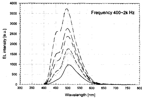
그림 6 인가 주파수 변화에 따른 발광 스펙트럼
