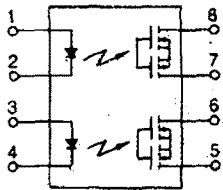
그림 3 무점접 광 릴레이(Nais, AQW214)
