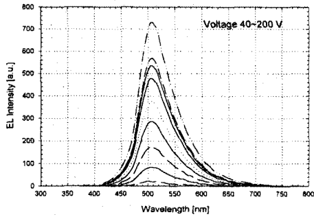
그림 5 인가 전압 변화에 따른 발광 스펙트럼
