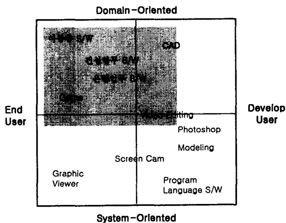
그림 1 소프트웨어 형태분류
