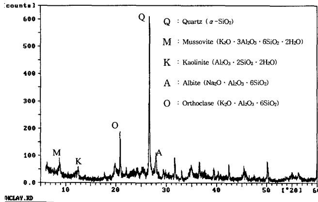
그림 1. 진해 해성점토의 XRD 분석결과
